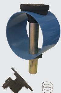
Membranens placering Membranen sidder i under ventilens låg
